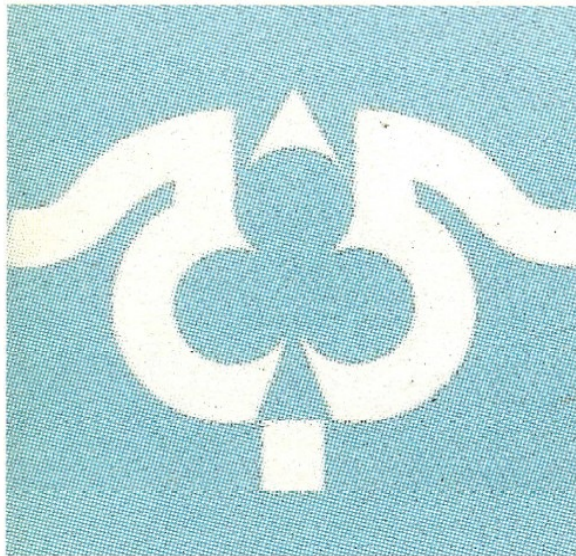
EEDF 1979_1984
